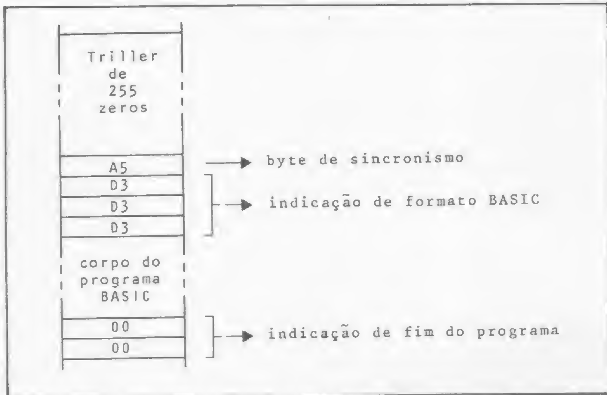
Figura 3 – Formato de uma fita BASIC.
